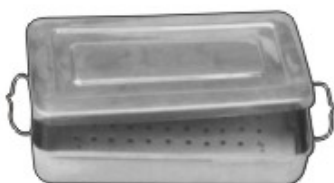
INSTRUMENT BOILER Size 15-240 180 x 80 x 40 mm 15-241 200 x 100 x 50 mm 15-242 250 x 125 x 40 mm 15-243 300 x 150 x 60 mm 15-244 350 x 175 x 75 mm 15-245 400 x 200 x 100 mm
